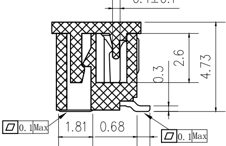
剖面 A-A
